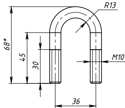
Поз.4 (Хомут)
