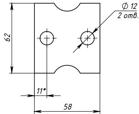
Поз.3 (Ушко) развертка
